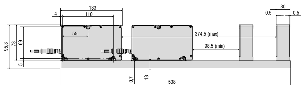
Source lumineuse et récepteur avec rail de montage
