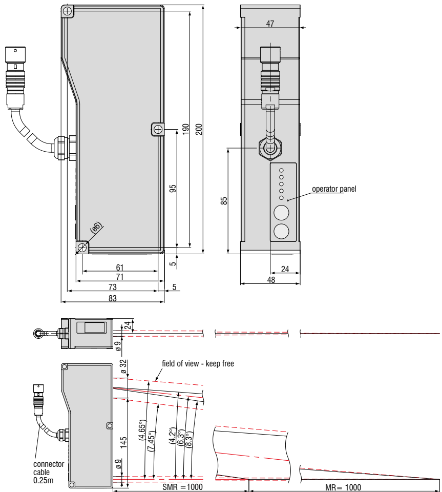
optoNCDT 1710-1000
