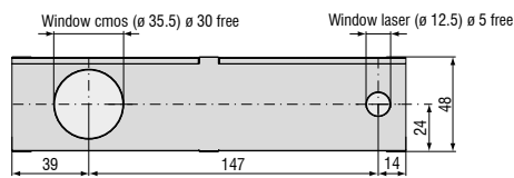
optoNCDT 1710-50 (50 mm)
